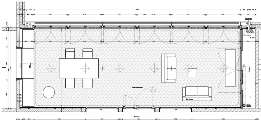
Grundriss (Moblierung)
