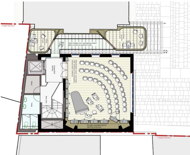
Grundriss 1. OG (Musikraum)
